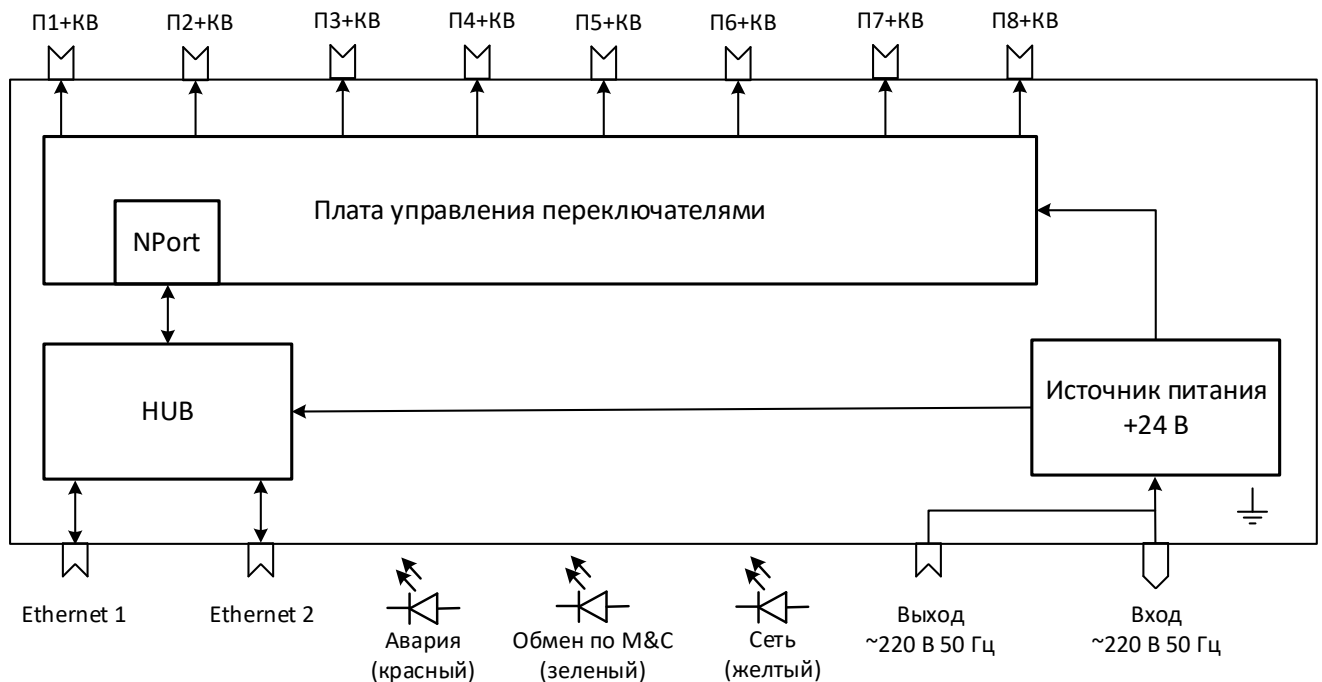
Рисунок 3 - Функциональная схема БУП 8-Х
